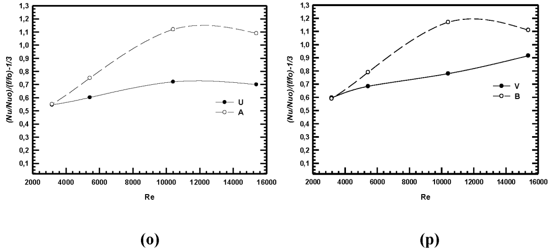
Şekil 4.15. (Devam) Isıl performans faktörünün Reynolds sayısı ile değişimi
