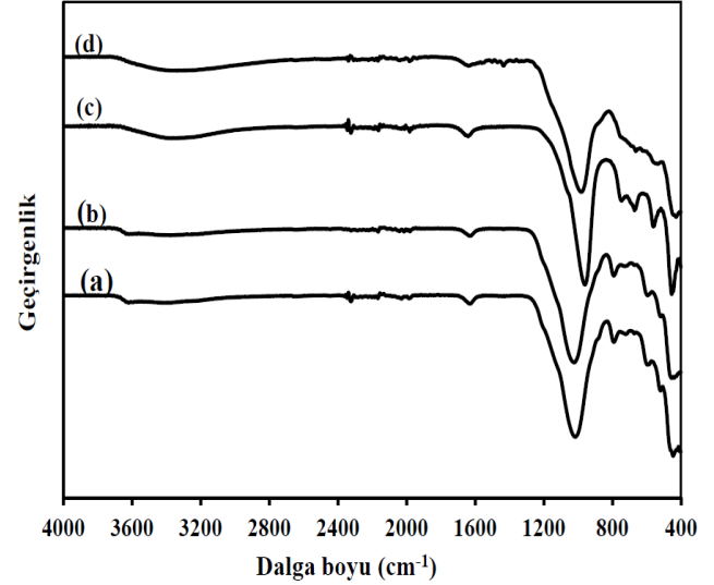
Şekil 2. FTIR spektrumları (a) Adsorpsiyon öncesi M-GZ (b) Adsorpsiyon sonrası M-GZ (c) Adsorpsiyon öncesi Z-10A (d) Adsorpsiyon sonrası Z-10A (The FTIR spectrums (a) Before adsorption M-GZ (b) After adsorption M-GZ (c) Before adsorption Z-10A (d) After adsorption Z-10A)
