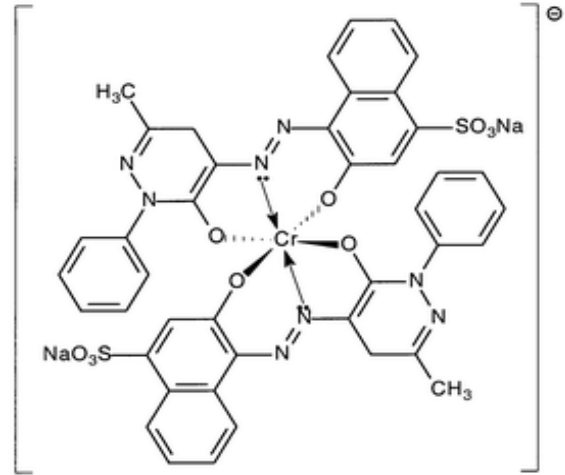
Şekil 1. C.I. Asit Viyole 90 (C.I. Acid Violet 90) [22]
